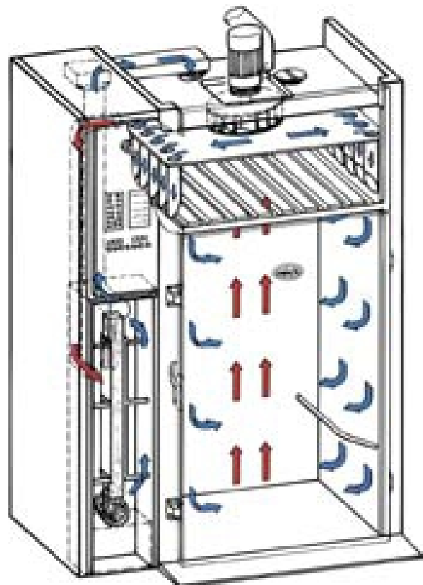
Das CIRCO-SYSTEM schematisch dargestellt
